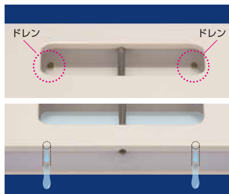
水抜き穴加工例
