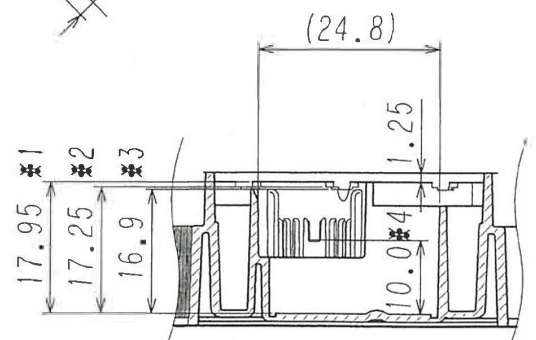
B-B断面図 (S=1/1)
