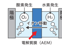
グリーン水素を製造するための電解質の構造
